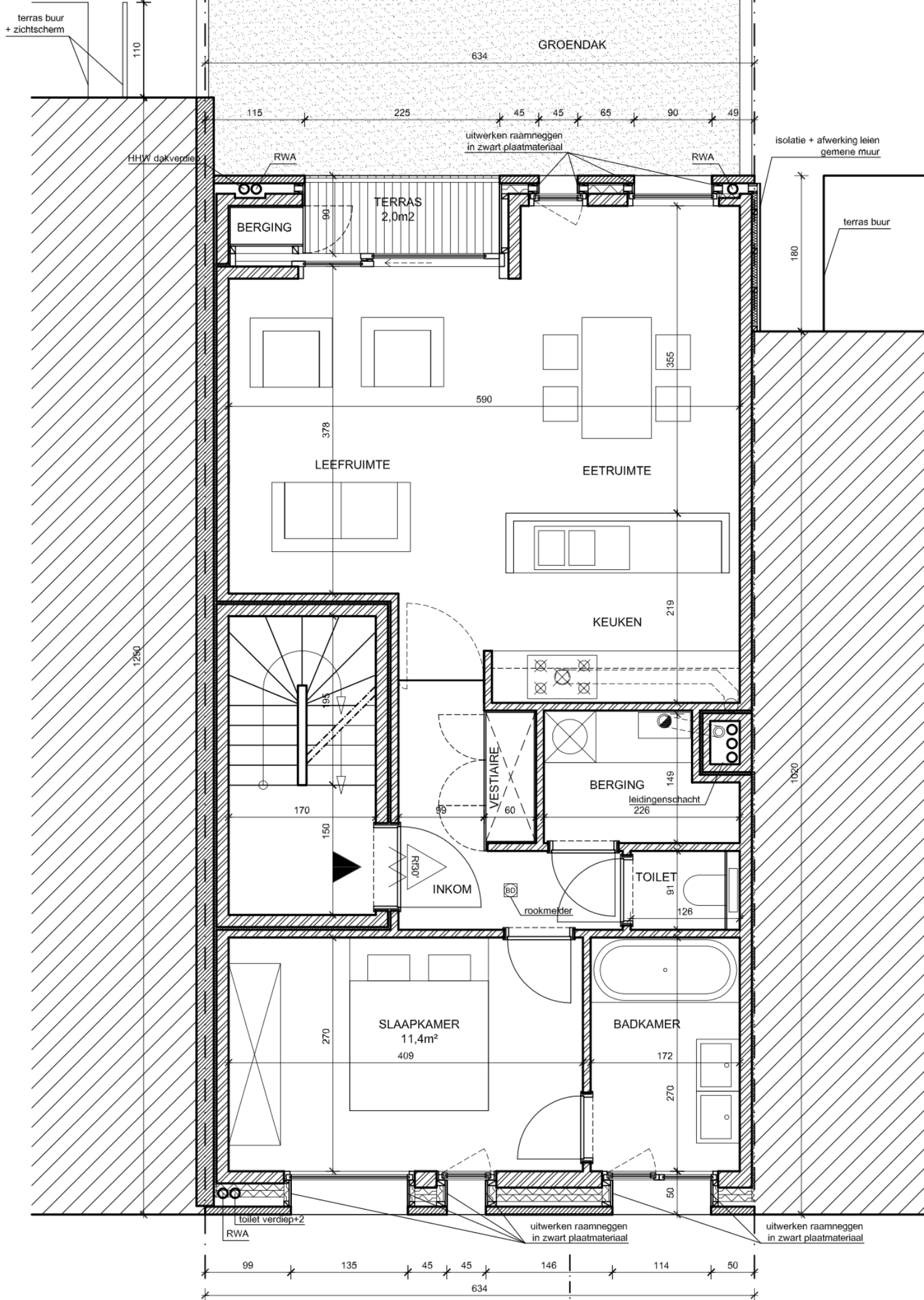
plan EERSTE VERDIEPING
